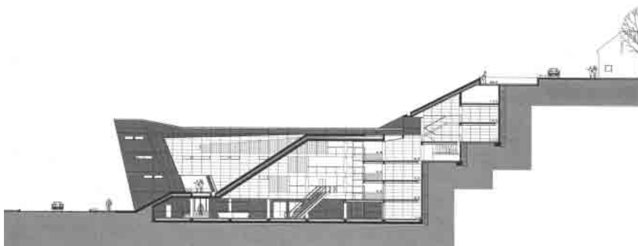
PRESEK 4-4 /KROZ HOL KULTURNOG CENTRA/
