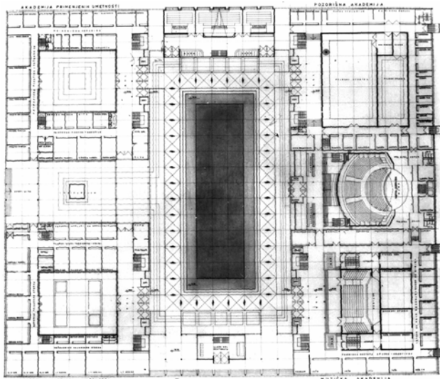
Konkurs za kompleks umetničkih akademija na Novom Beogradu, Otkup (L.Lenarčić, M.Mitić, I.Petrović, M.Čanak), Za naše uslove neuobičajeno blok-rešenje sa centralnim atrijumom.
