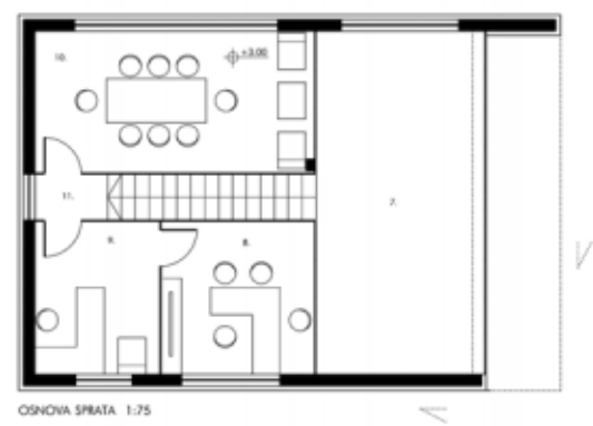
OSNOVA SPRETA 1:75
