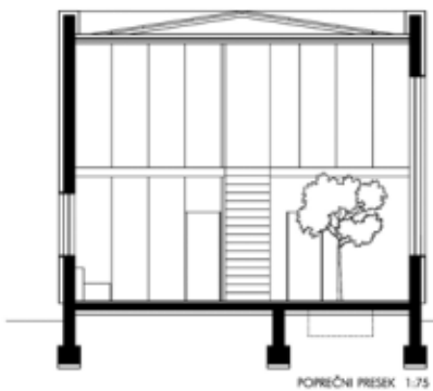
POPREČNI PRESEK 1:75
